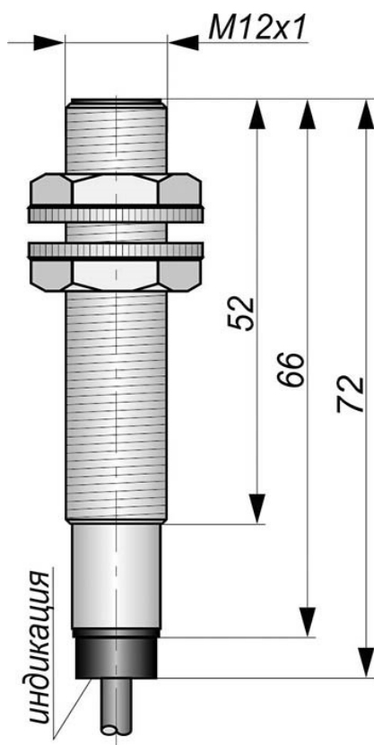
Габаритный чертеж
