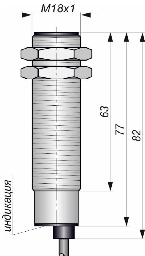
Габаритный чертеж
