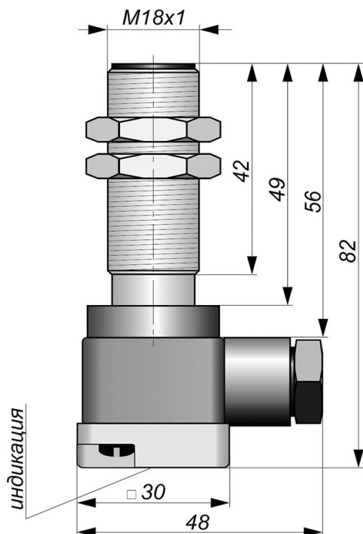
Габаритный чертеж
