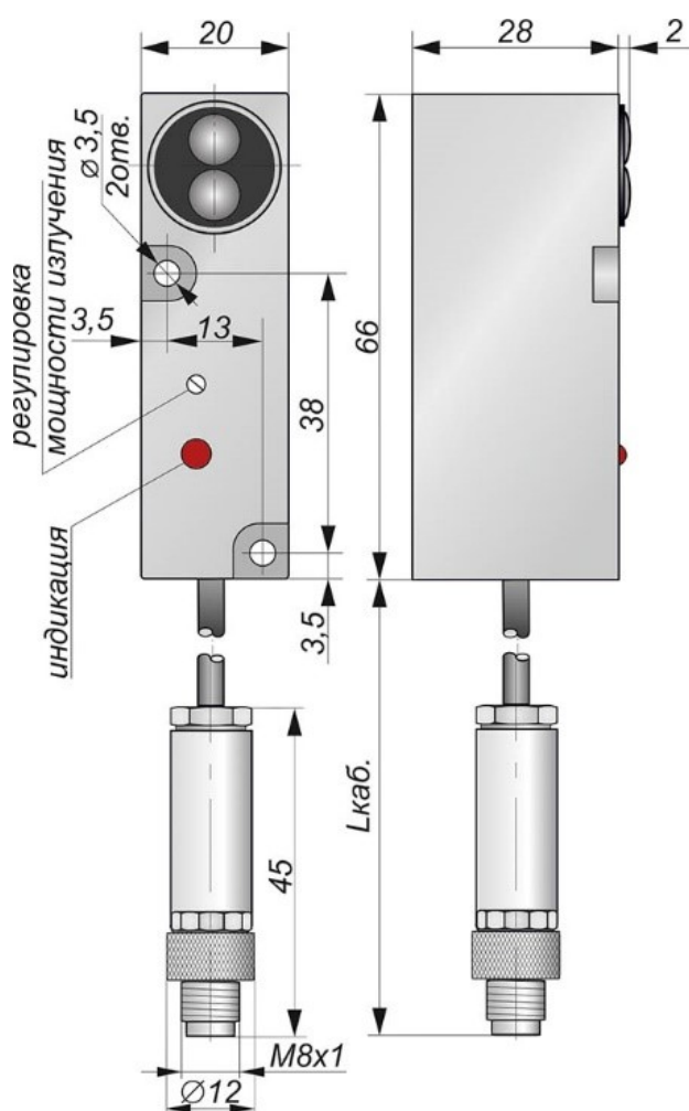
Габаритный чертеж
