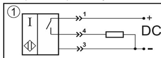
Цоколевка разъема
