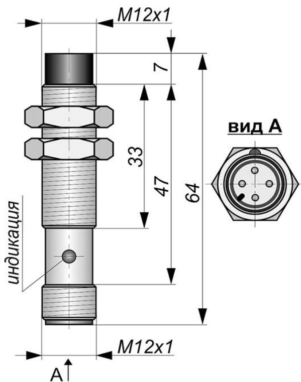
Габаритный чертеж
