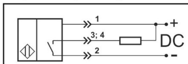
Цоколевка разъема
