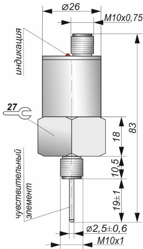
Габаритный чертеж
