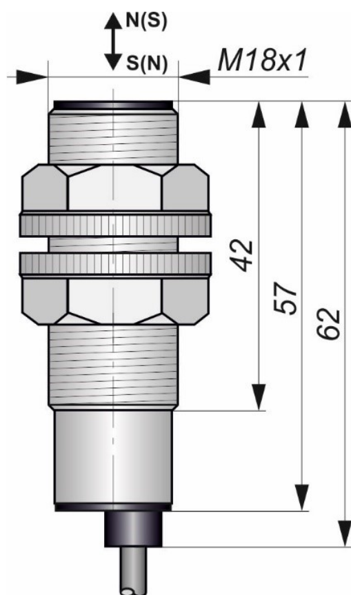
Габаритный чертеж
