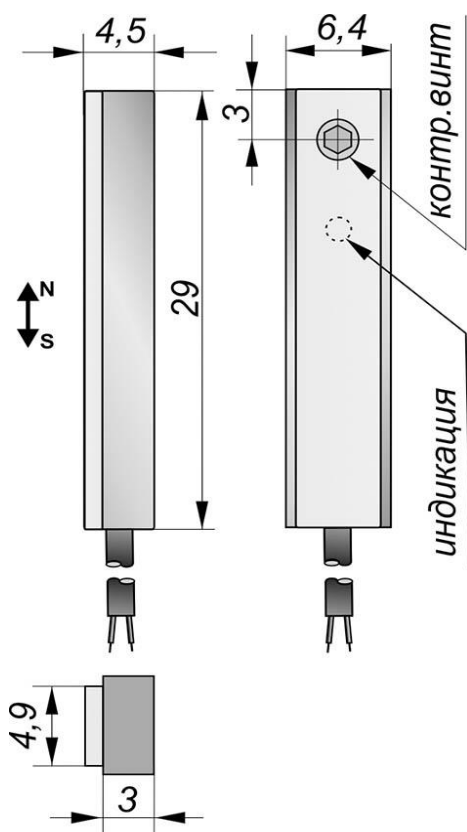
Габаритный чертеж
