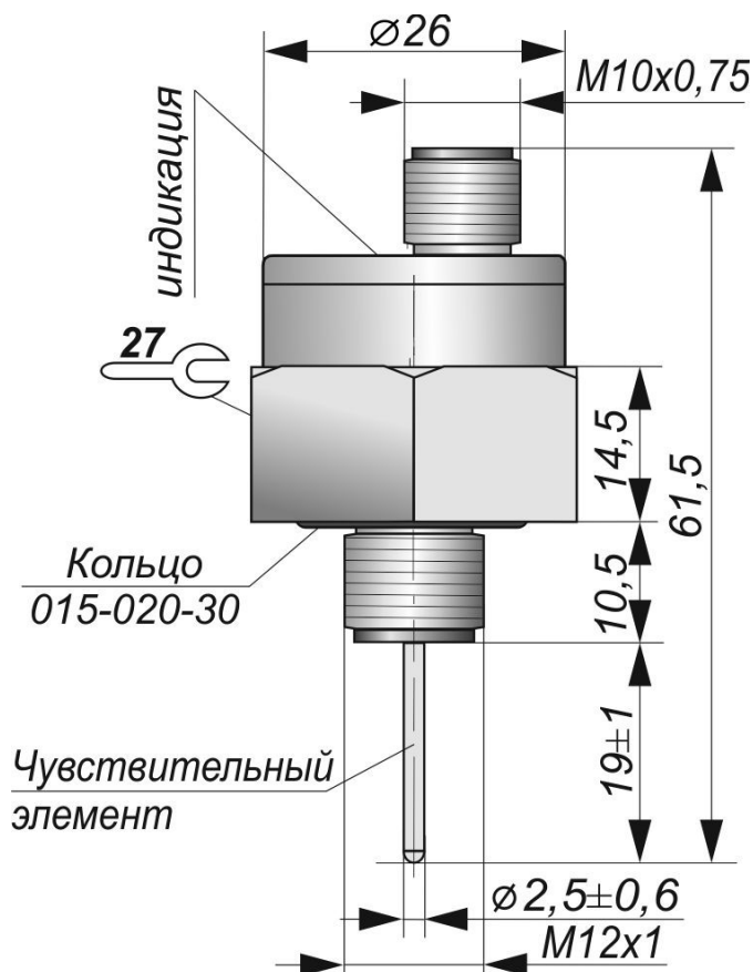
Габаритный чертеж
