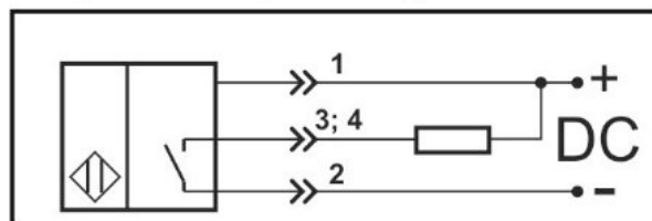
Цоколевка разъема
