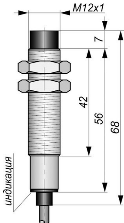
Габаритный чертеж
