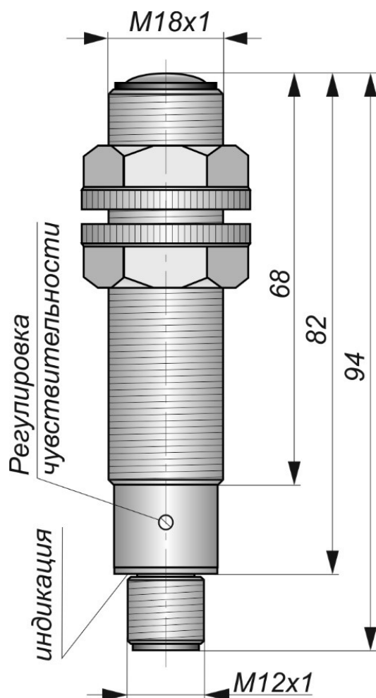
Габаритный чертеж
