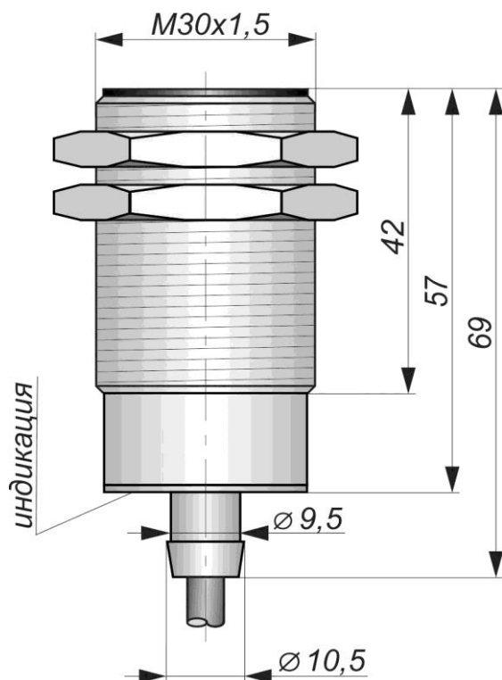
Габаритный чертеж
