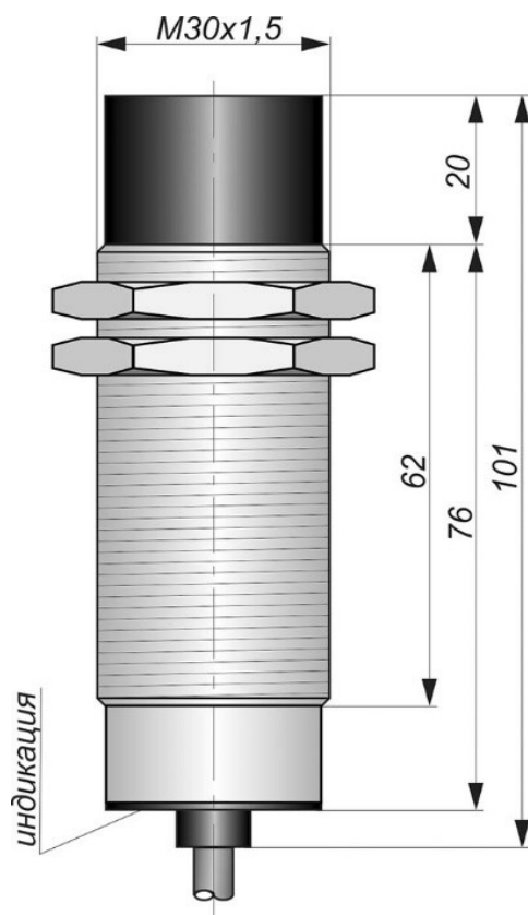
Габаритный чертеж
