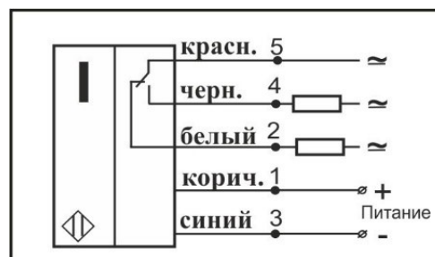
Схема соединения
