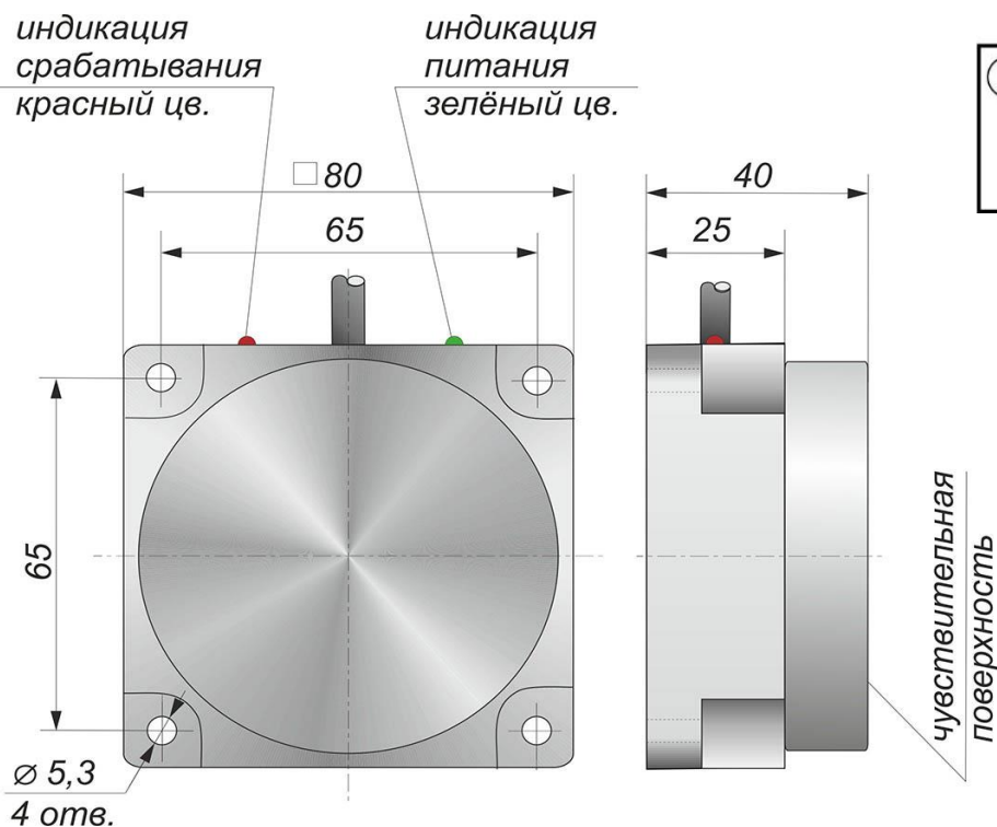
Габаритный чертеж
