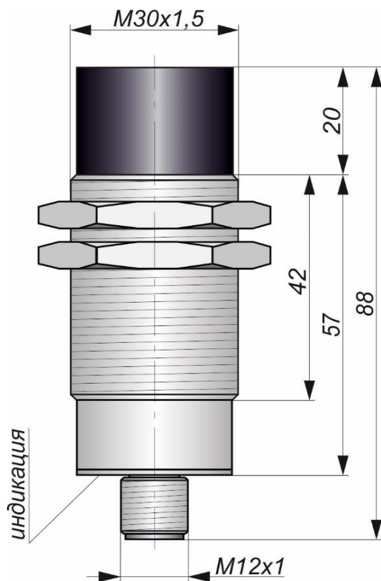
Габаритный чертеж
