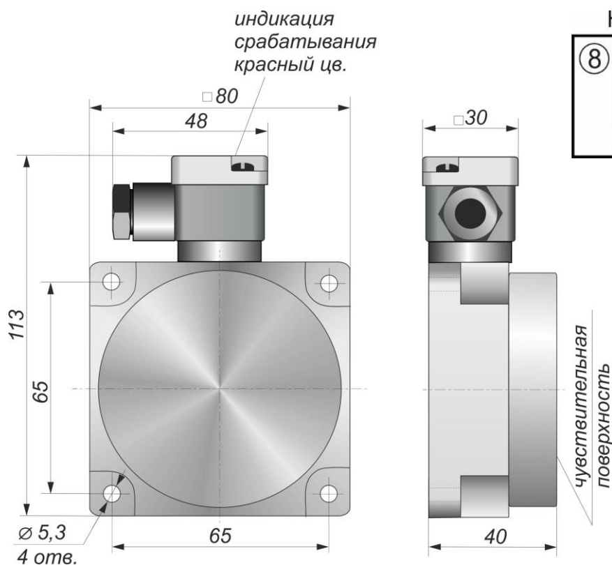
Габаритный чертеж
