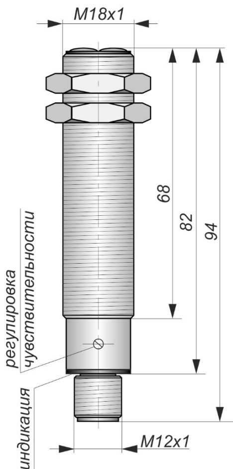
Габаритный чертеж
