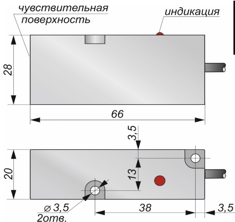
Габаритный чертеж
