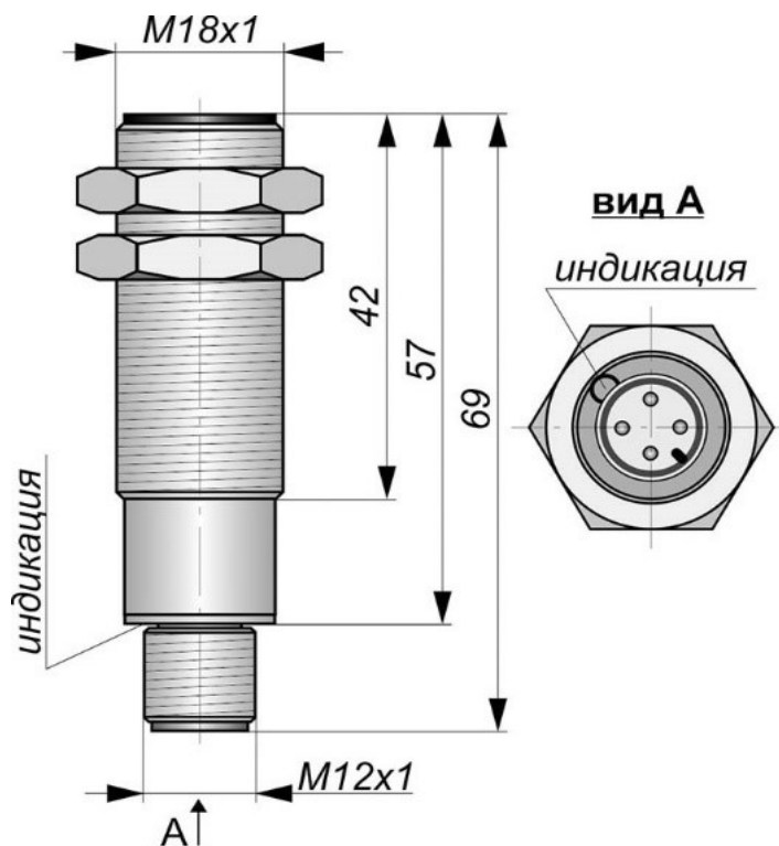
Габаритный чертеж
