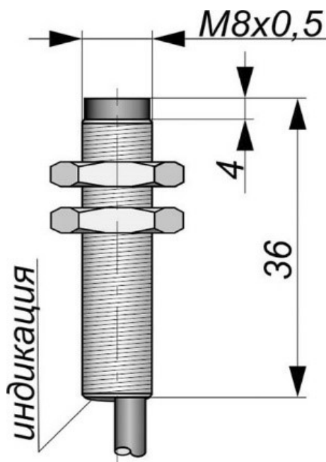
Габаритный чертеж
