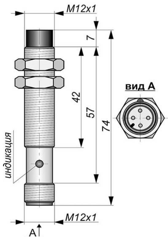
Габаритный чертеж
