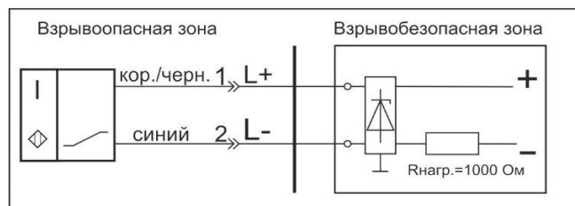
Схема соединения
