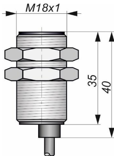
Габаритный чертеж
