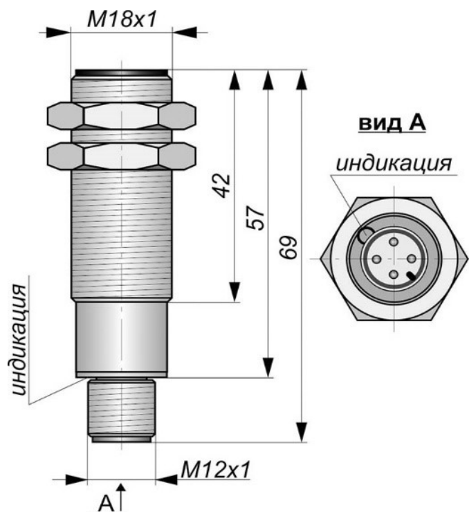
Габаритный чертеж
