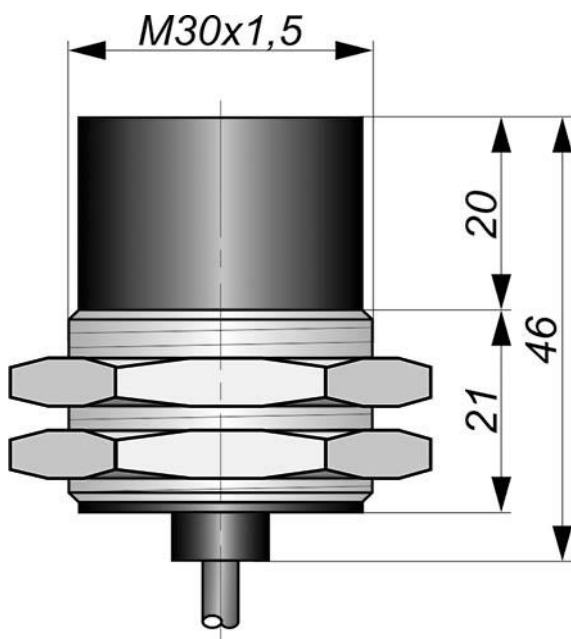
Габаритный чертеж
