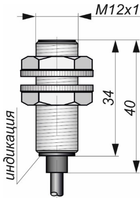
Габаритный чертеж
