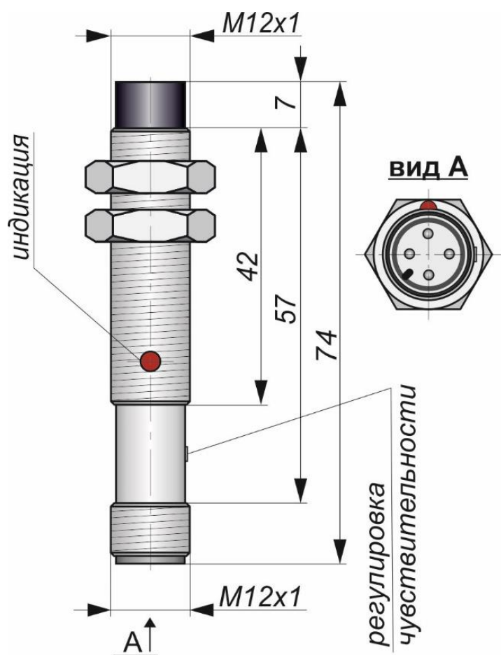
Габаритный чертеж
