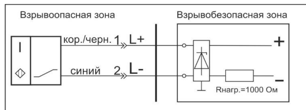
Схема соединения
