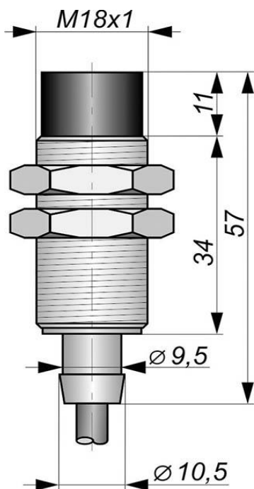
Габаритный чертеж
