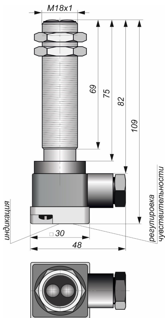
Габаритный чертеж
