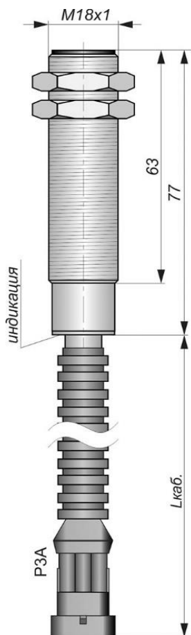
Габаритный чертеж
