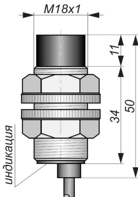
Габаритный чертеж
