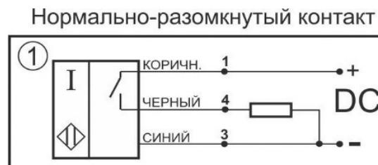
Схема соединения
