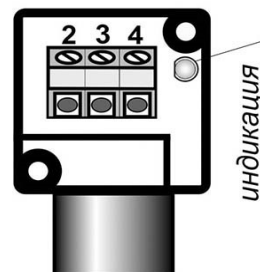
Цоколевка клеммной колодки
