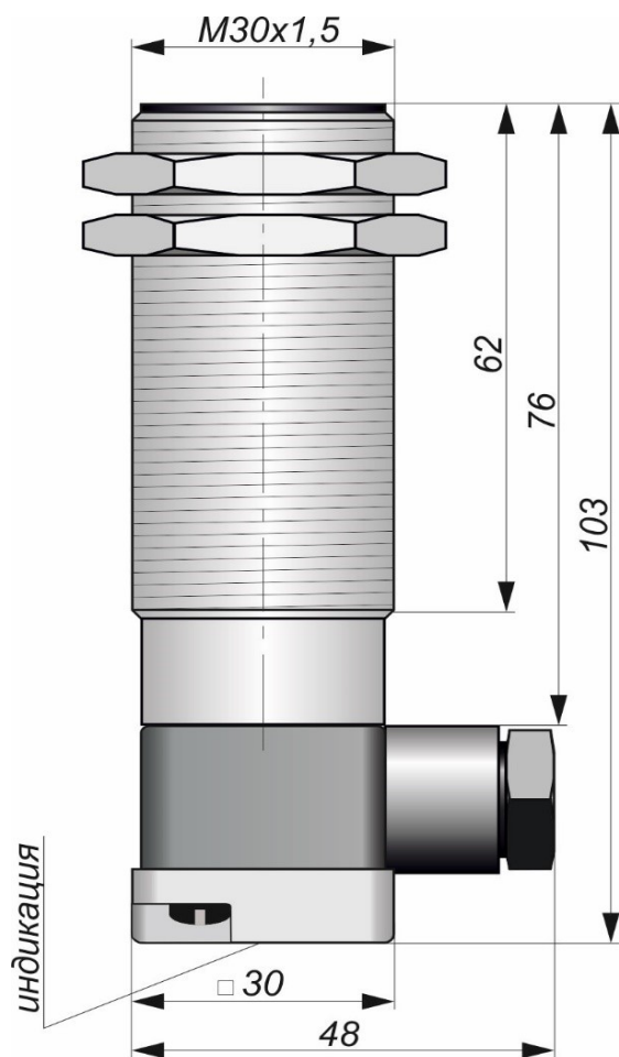
Габаритный чертеж
