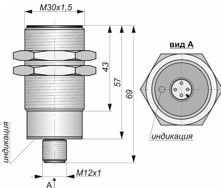
Габаритный чертеж
