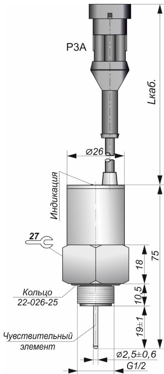
Габаритный чертеж
