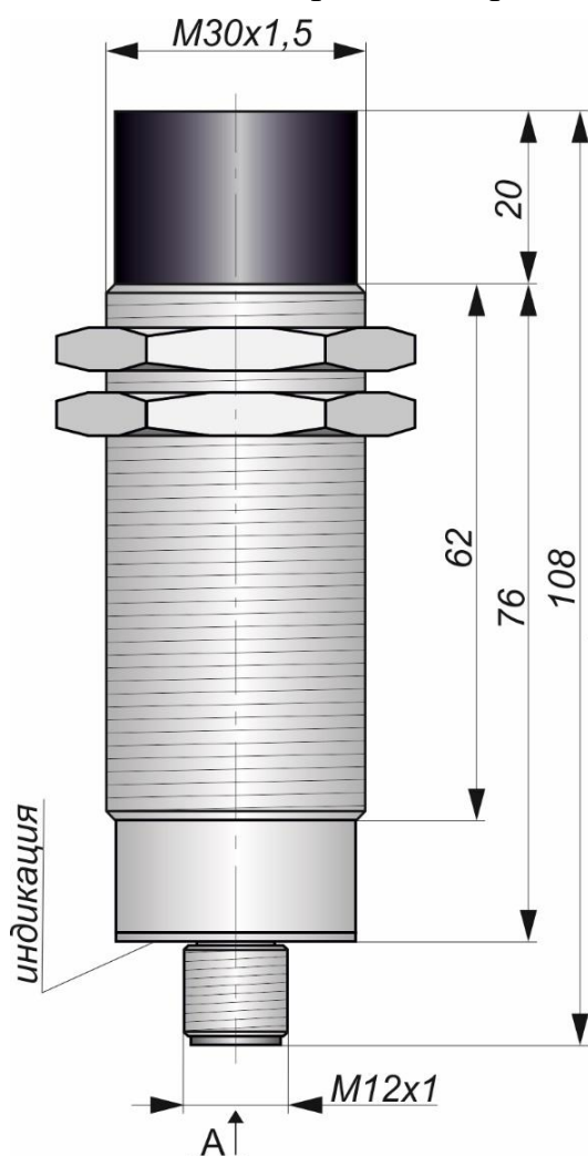
Габаритный чертеж
