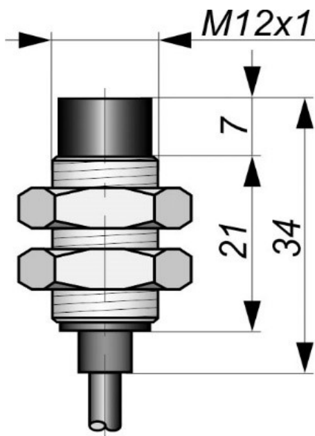
Габаритный чертеж
