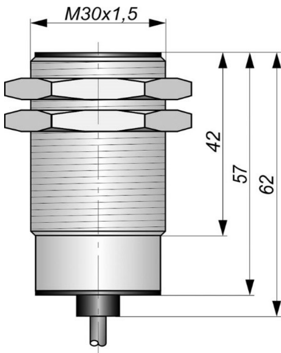
Габаритный чертеж
