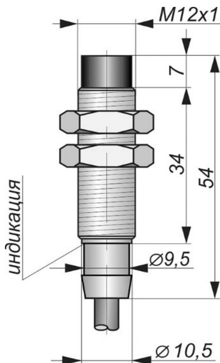
Габаритный чертеж
