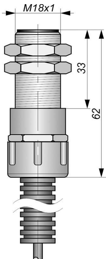
Габаритный чертеж
