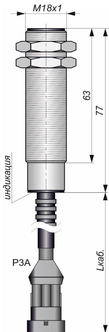
Габаритный чертеж
