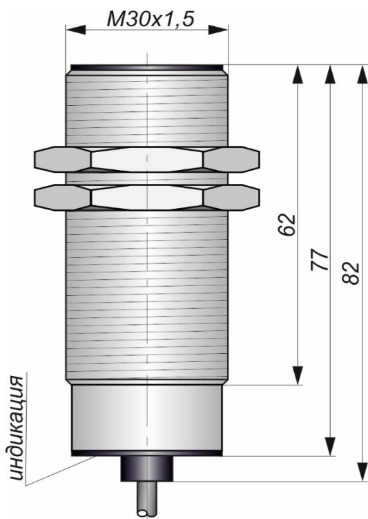
Габаритный чертеж
