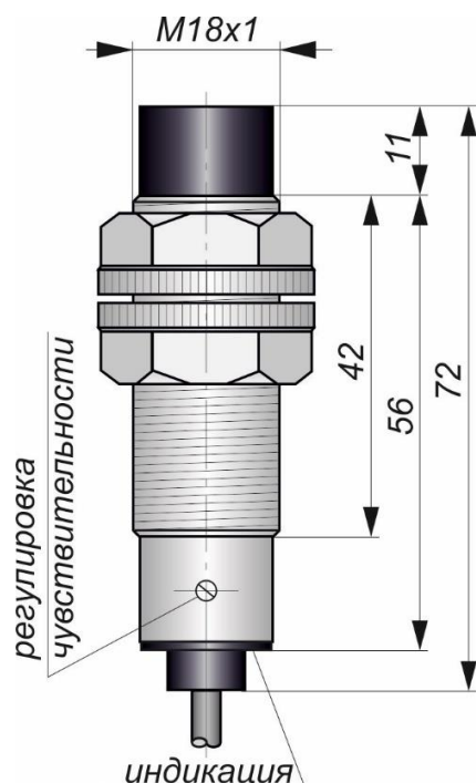
Габаритный чертеж
