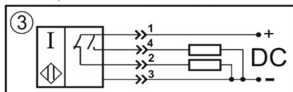
Переключающий контакт
