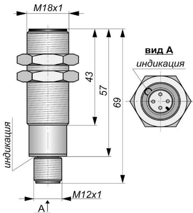
Габаритный чертеж
