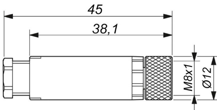
Габаритный чертеж
