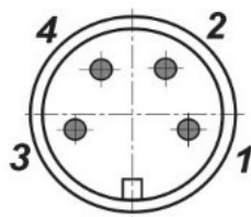
Цоколевка разъема
