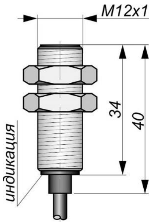
Габаритный чертеж
