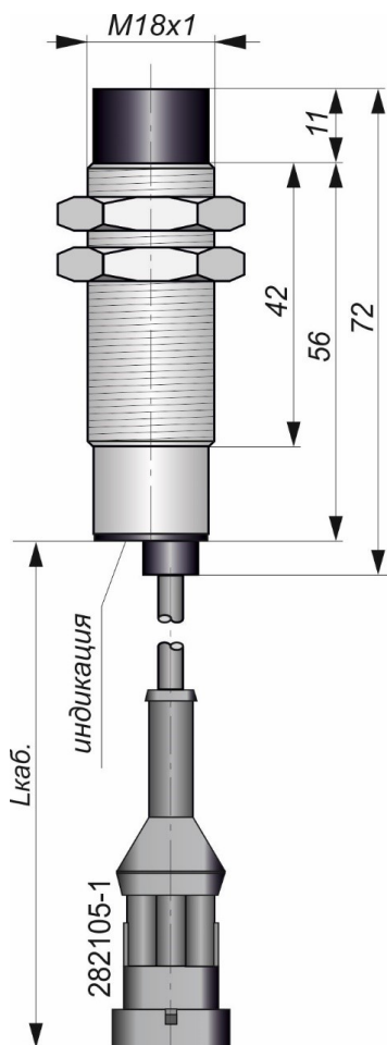
Габаритный чертеж
