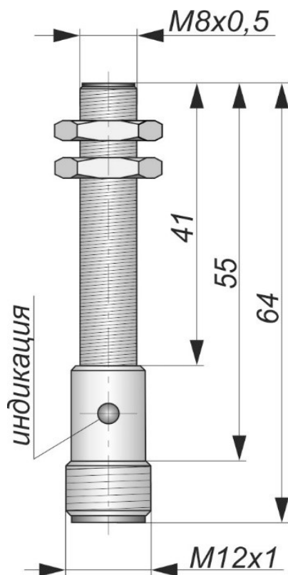
Габаритный чертеж
