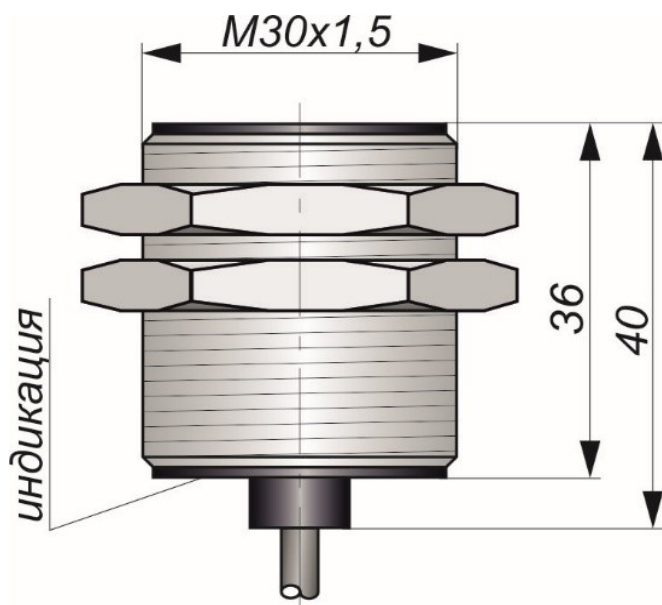
Габаритный чертеж
