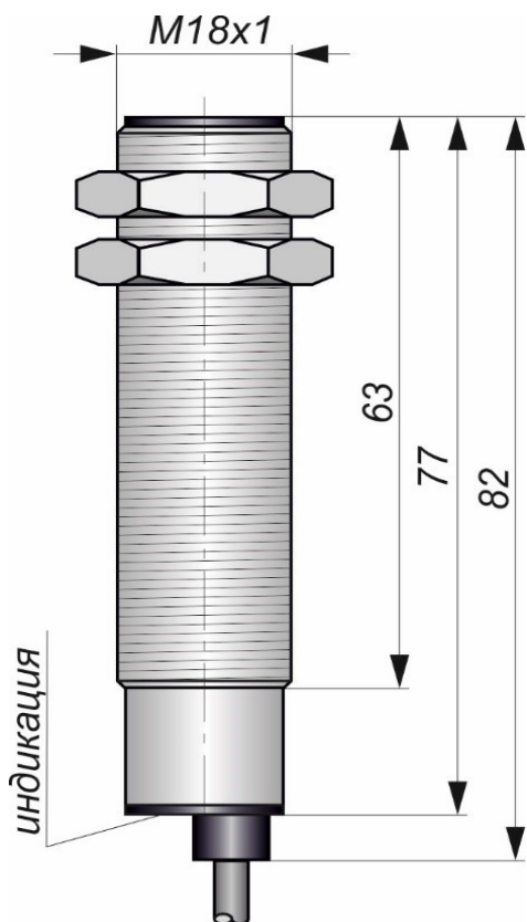
Габаритный чертеж
