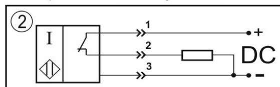
Нормально-замкнутый контакт
