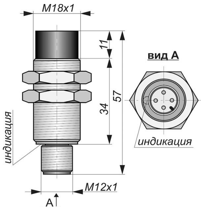
Габаритный чертеж
