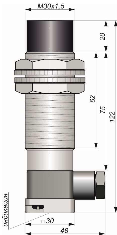
Габаритный чертеж
